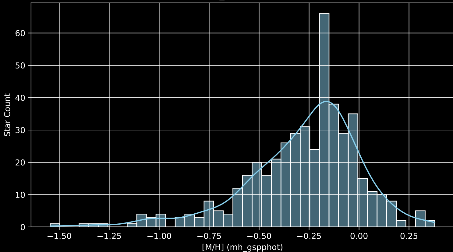
GALAH DR4 Field: [6776] [M/H] (mh_gspphot) (n= 459)
