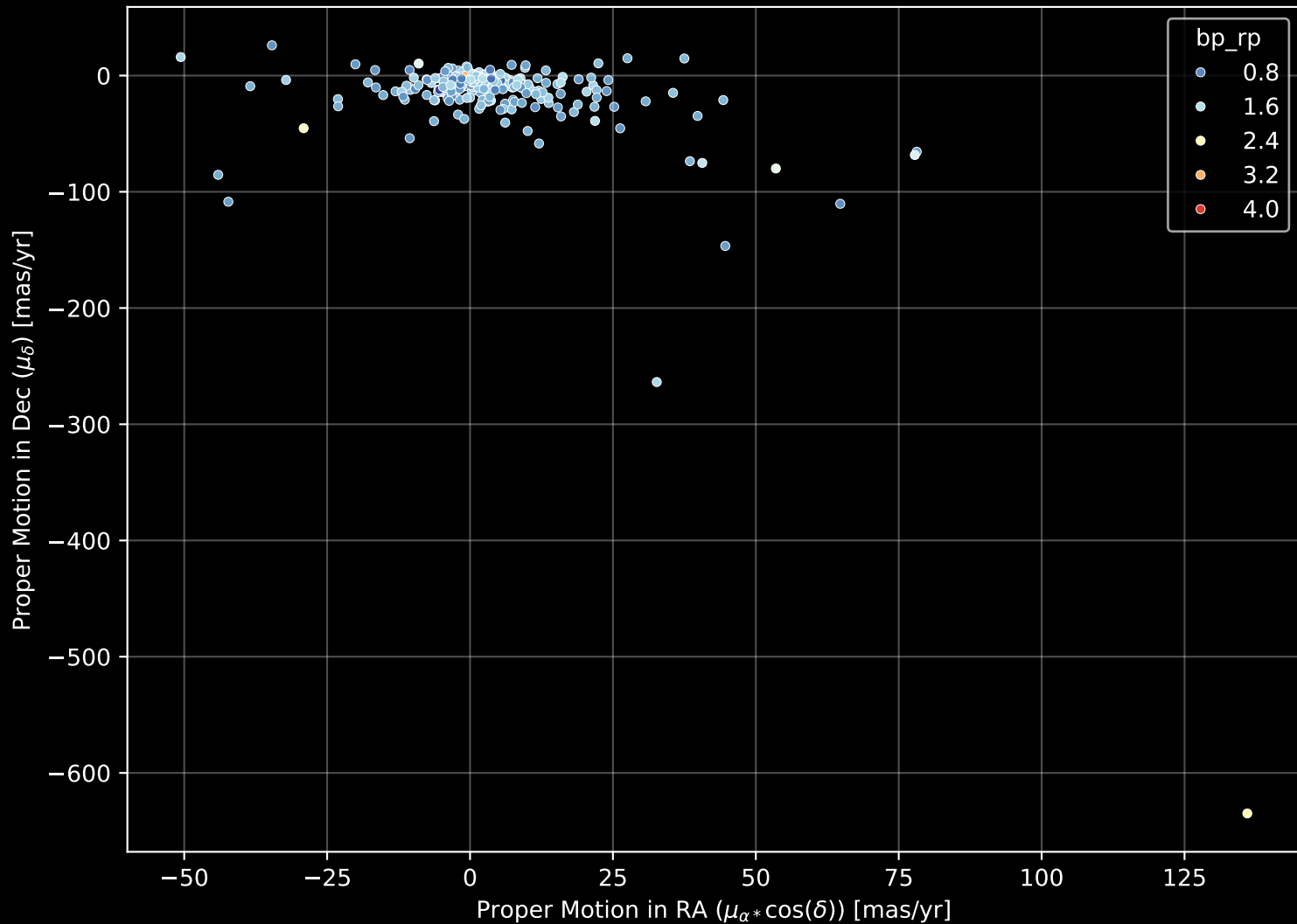
GALAH DR4 Field: [6776] Proper Motion Diagram (n= 461)
